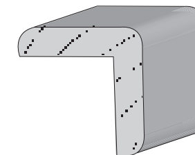
EC205 Corner 1-1/16" x 1-1/16"
